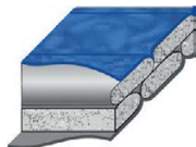
2-х слойная конструкция наполнителя
